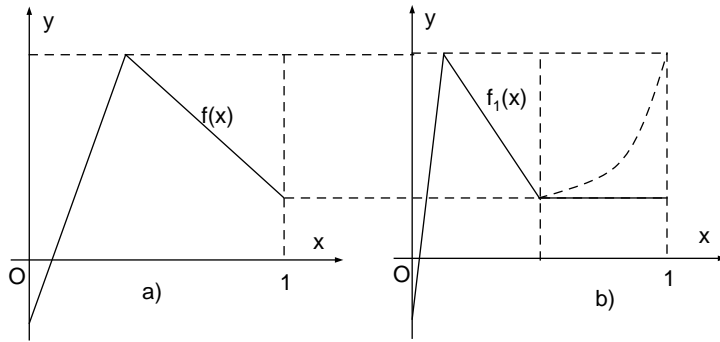
рис. 11.1. Деформация бесконечномерной сферы
