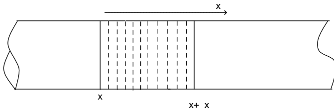
рис. 14.2. Распространение сжатия
