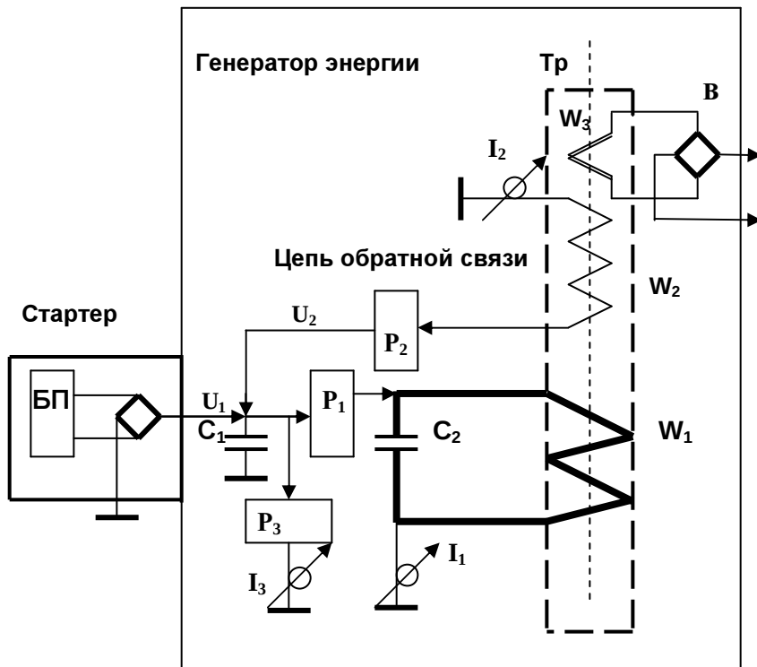
Рис. 19. Вариант блок-схемы макета для получения энергии из эфира: БП – блок питания; Тр – трансформатор; W_1 – первичная катушка трансформатора; W_2 – катушка обратной связи; W_3 – выходная катушка трансформатора; C_1 – зарядная емкость питания; C_2 – емкость контура (не установлено, нужна ли она); P_1 – разрядник прямой связи ( U_1 пробоя порядка 1 кВ/мм); P_2 – разрядник (или диод) обратной связи ( U_2 > U_1 ); P_3 – разрядник (или схема) ограничения напряжения ( U_3 > U_2 ); I_1 – ток в цепи первичной обмотки трансформатора; I_2 – ток в цепи обратной связи; В – выход.
