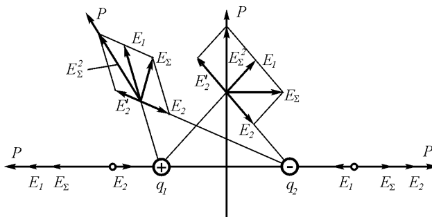
Рис. 5.9. Излучение энергии диполем с сосредоточенными параметрами
