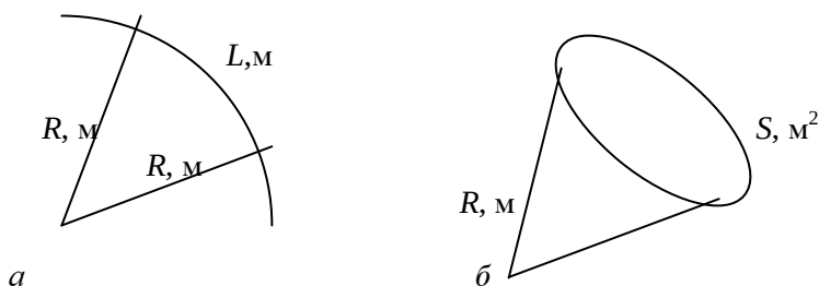
Рис. 1.1. К определению размерностей радиана (а) истерадиана (б)
