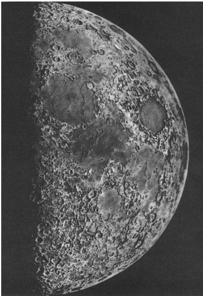
Рис. 5.9. Поверхность Луны в первой четверти (по рисунку чешского астронома И.Клепшты)
