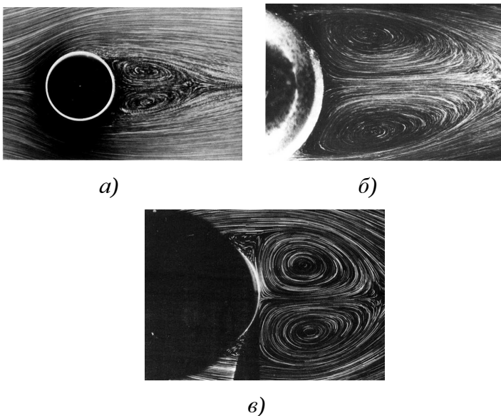
Рис. 6.5 Обтекание тела вращения потоками газа: a — обтекание кругового цилиндра при Re = 26 ; б — обтекание шара при Re = 118 ; в — обтекание шара при Re = 500
