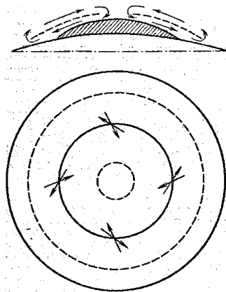
Рис. 6.6.Схема циркуляции воздуха над Антарктидой
