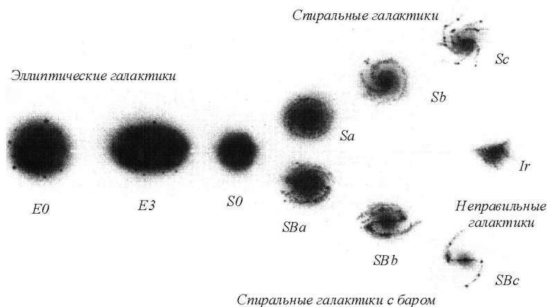
Рис. 4.4. Морфологическая классификация галактик по Хаббл: различные типы галактик расположены на схеме таким образом, что относительное содержание в них газа и молодых звезд уменьшается слева направо.
