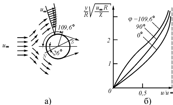
Рис. 7.14. Обтекание шара газовым потоком: а – направление потоков; б – эпюра изменения относительной скорости потока с увеличением расстояния от поверхности шара
