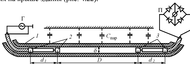
Рис. 4.22. Схема эксперимента по проверке продольного распространения излучения диполя с сосредоточенными параметрами: 1 – резиновый шланг, наполненный подсолонной водой; 2 – электроды излучающего диполя; 3 – электроды приемного диполя
