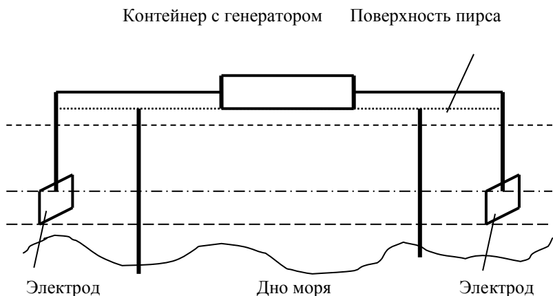
Рис. 4.25. Схема расположение генератора на пирсе
