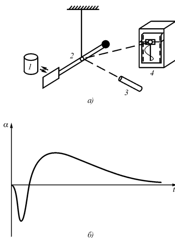
Рис. 3.21. Схема лабораторного эксперимента по выявлению лептонной пены при образовании ковалентной химической связи (а) и график отклонения паруса весов при проведении химической реакции (б): 1 – стаканчик с химическими реактивами; 2 – крутильные весы; 3 – лазер; 4 – самописец.
