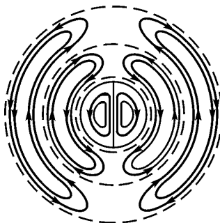
Рис. 2.9. Вихрь Тэйлора
