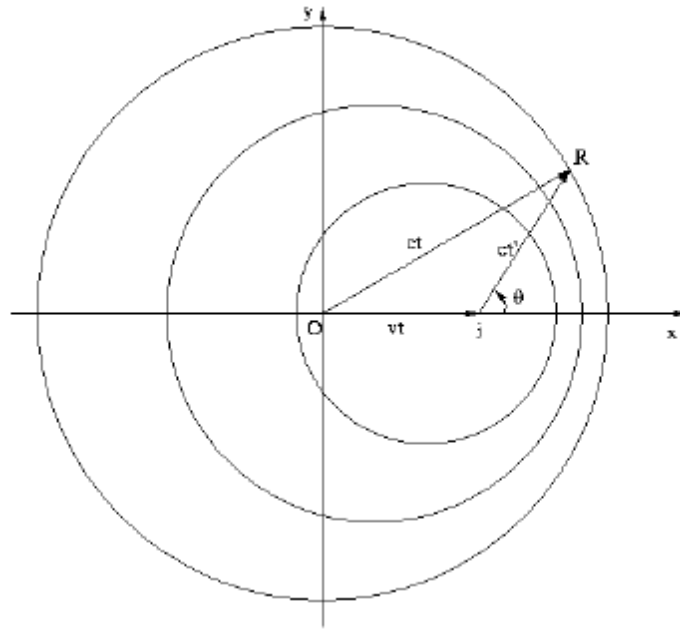
図 3.5. 波源が運動しているときのドップラー効果
