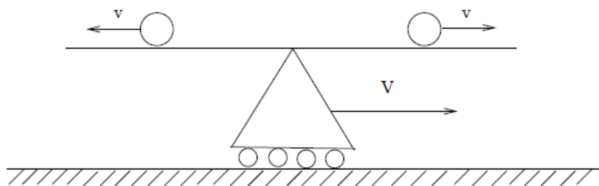
図 1.27. 速度合成則と天秤の矛盾
