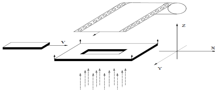
図 1.23. 棒の「方向転換」
