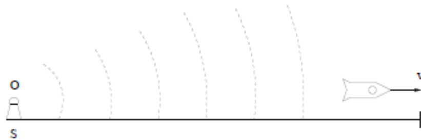
図 1.12. 固有時間信号の交換
