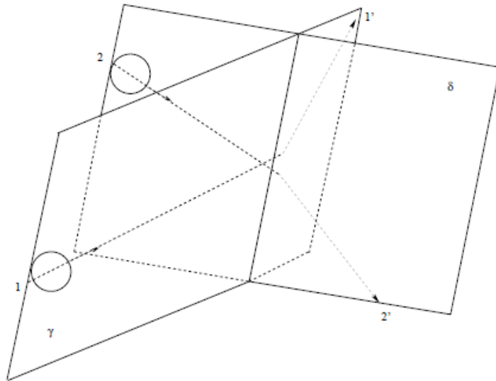
図 4.9. 2つの粒子の衝突の三次元性
