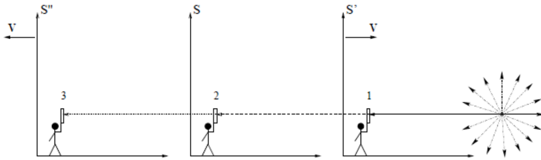
図 1.16. 同時性の相対性の矛盾
