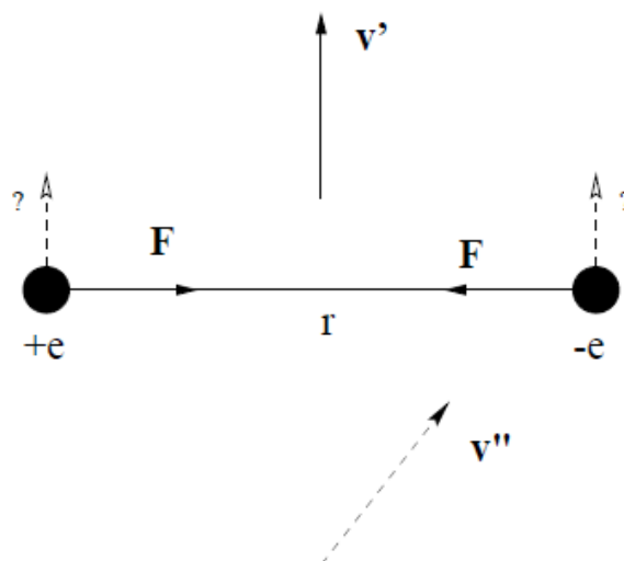
図 4.2. 平行に飛行する 2 つの電荷
