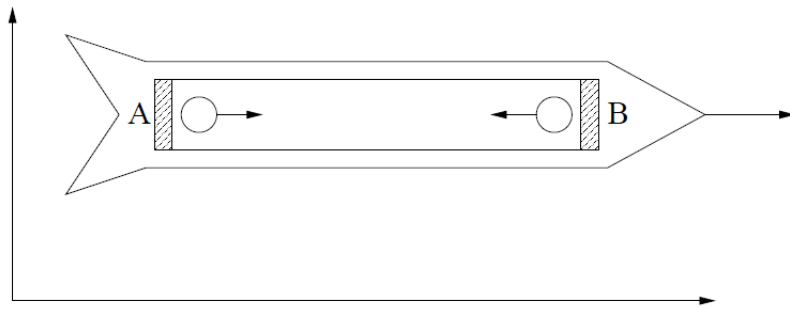
図 4.1. 砲丸の入った管の質量中心
