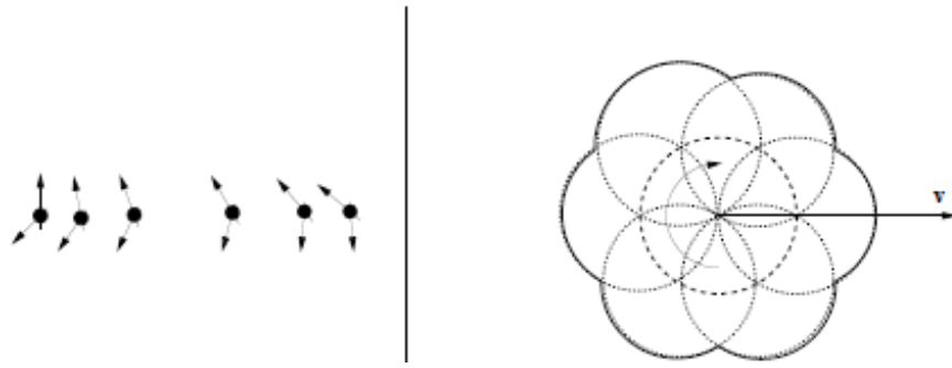
図 D.2. 光のモデル
