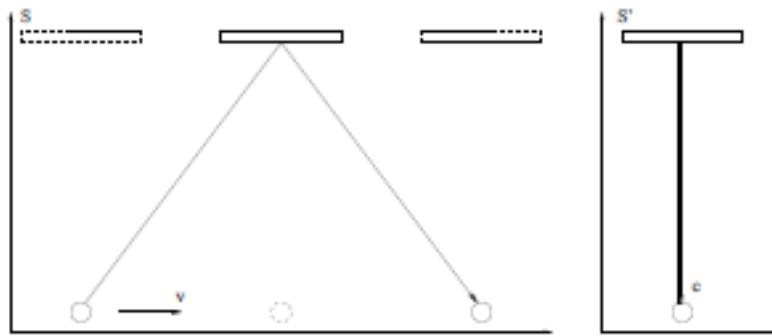
図 1.14. 光時計
